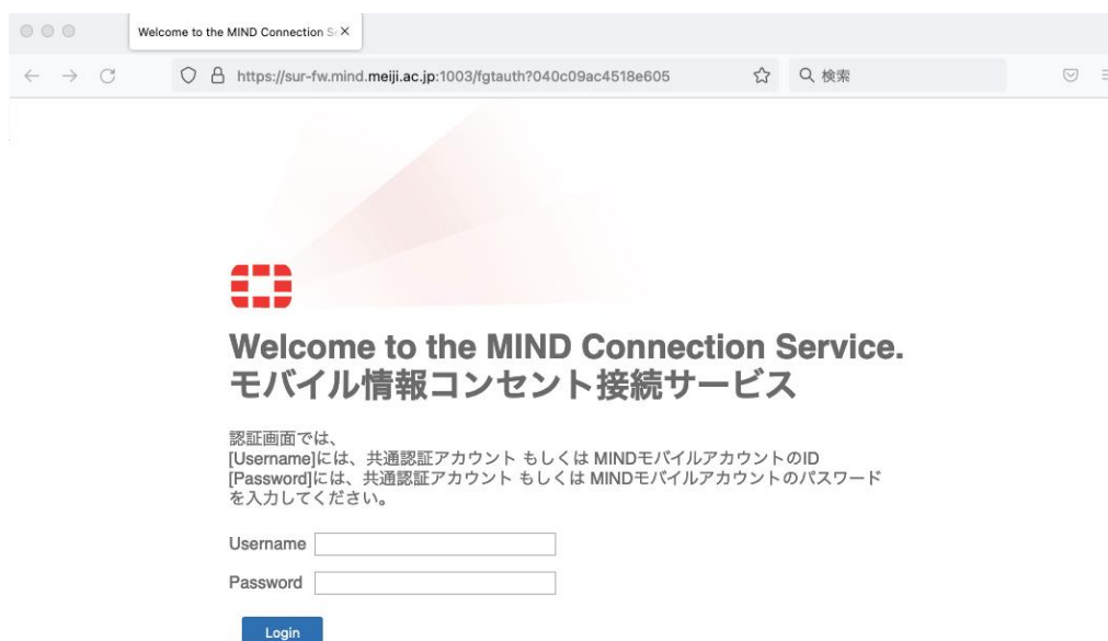
(図3-1) 「認証画面」
