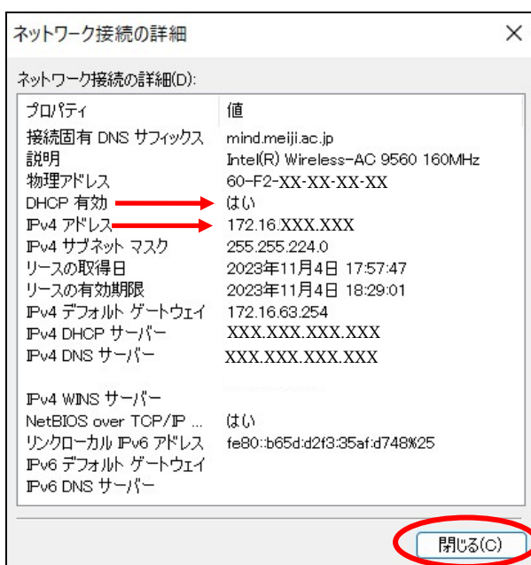
図 3-6 「ネットワーク接続の詳細」ウィンドウ
