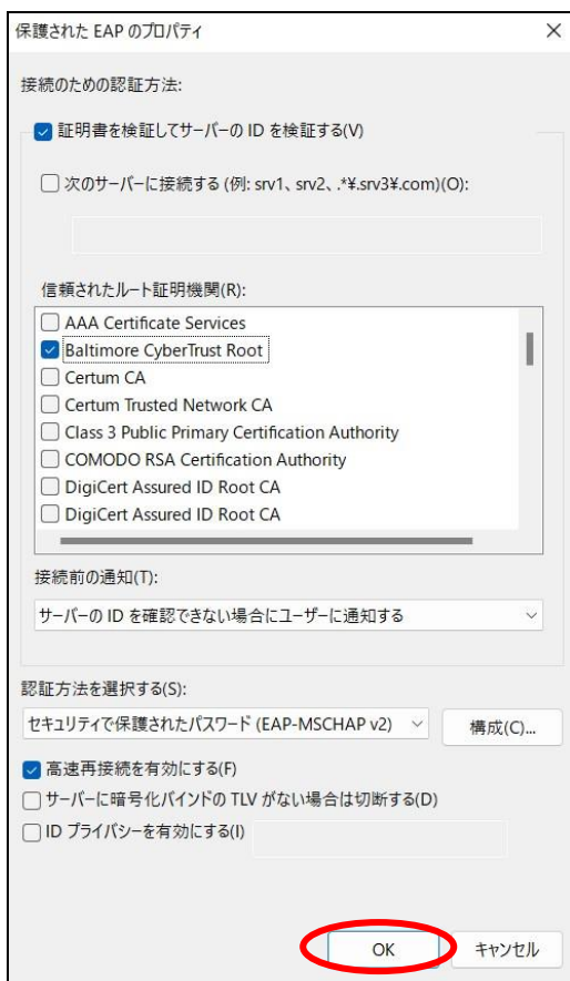
図 1-2-12 「保護された EAP のプロパティ」 の画面
